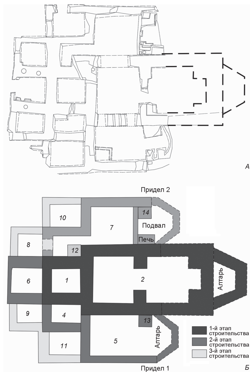
Рис. 4. Предварительная реконструкция фундамента.
